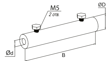
Зажим продольный
