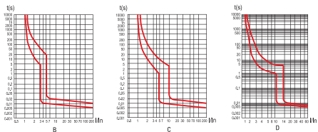
Рис. 1 Время-токовые характеристики
