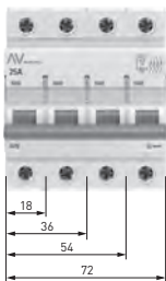
Габаритные размеры выключателей нагрузки AVN серии AVERES для номиналов 25 А, 40 А, 63 А
