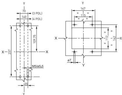
Шаблон для разметки сверления металлической панели
