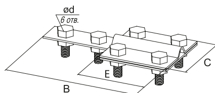
Зажим контрольный
