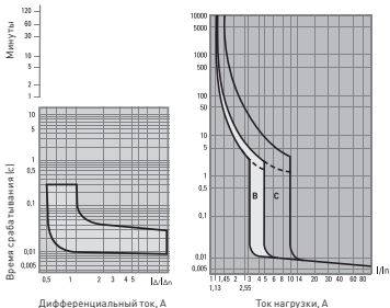
Рис. 1 - Время-токовые характеристики
