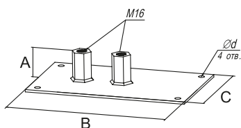
Подставка 1–4 метров
