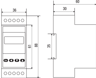
Рис. 2 Габаритные размеры
