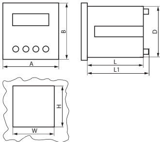
Рис. 2 Габаритные размеры
