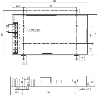
Рис 5. Габаритные размеры (MPS-200W-24, MPS-350W-24)
