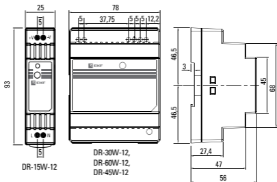
Рис. 2 Габаритные размеры блока питания.
