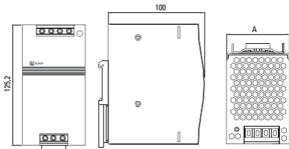
Рис. 3 Габаритные размеры блока питания DR-75W-12, DR-120W-12.
