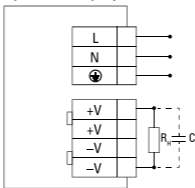
Рис. 1 Схема подключения блока питания
