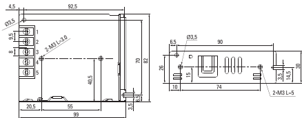
Рис 1. Габаритные размеры (MPS-35W-24, MPS-50W-24)
