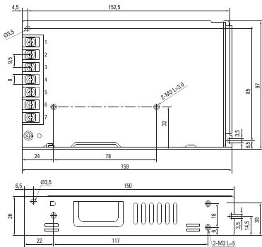
Рис 4. Габаритные размеры (MPS-150W-24)
