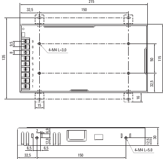
Рис 5. Габаритные размеры (MPS-200W-24, MPS-350W-24)
