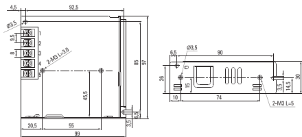
Рис 2. Габаритные размеры (MPS-75W-24)
