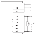
Рис 8. Схема подключения (MPS-200W-24, MPS-350W-24)
