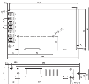
Рис 4. Габаритные размеры (MPS-150W-24)
