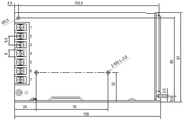
Рис 3. Габаритные размеры (MPS-100W-12)
