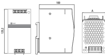
Рис. 3 Габаритные размеры блока питания DR-75W-12, DR-120W-12.
