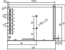
Рис 3. Габаритные размеры (MPS-100W-12)
