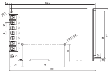
Рис 3. Габаритные размеры (MPS-100W-24)
