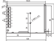
Рис 3. Габаритные размеры (MPS-100W-24)
