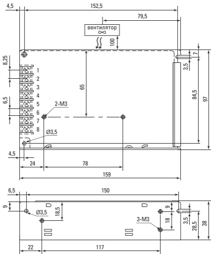
Рис 1. Габаритные размеры MPSu-55W-24
