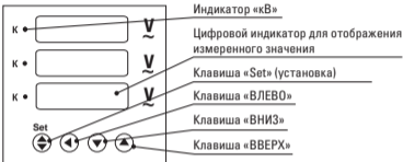
Рис.1 Лицевая панель прибора
