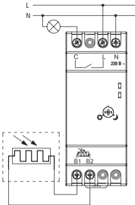
Рис.3 Схема подключения фотореле DIN-1 (ФР)
