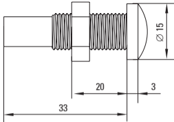
Рис.2 Габаритные размеры датчика освещенности
