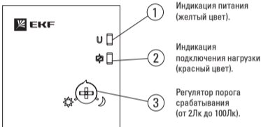
Рис.4 Назначение органов управления и индикации
