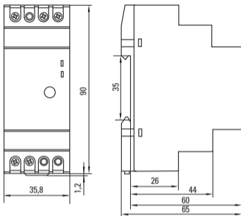
Рис.1 Габаритные размеры фотореле DIN-1 (ФР)
