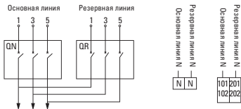
Схема соединения 4-х полюсного АВР
