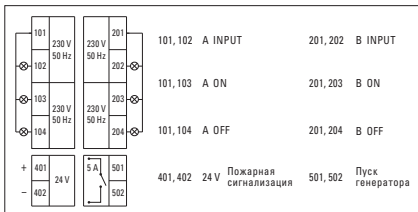
Присоединение контрольных проводников к контроллеру:
