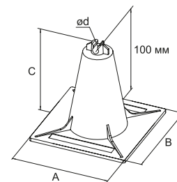
Держатель для мягкой кровли
