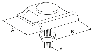
Зажим (полоса-прут)
