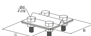
Зажим (полоса-прут)
