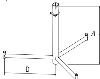
Тренога
