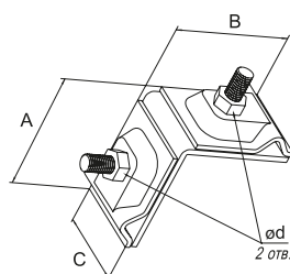
Держатель фальцевый
