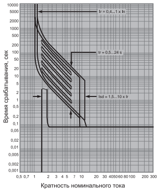
Время-токовые характеристики ВА-99С 1250
