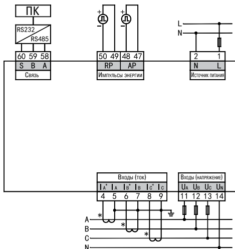
Рис. 4 Расположение клемм
