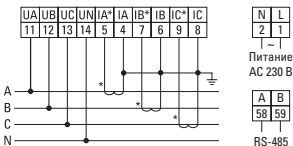
Рисунок 6 – Схема подключения прибора DMC-r
