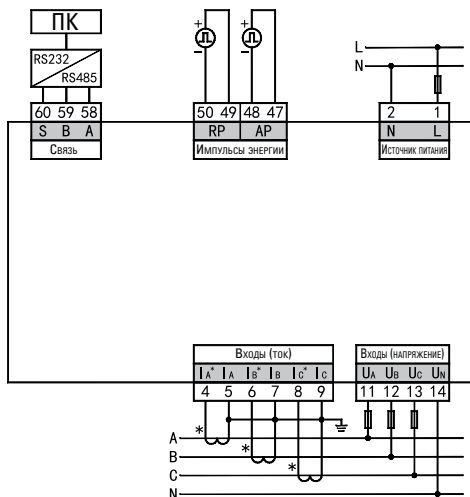
Рис. 4 Расположение клемм
