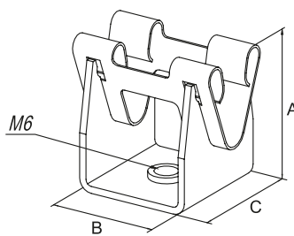
Держатель токоотвода металлический
