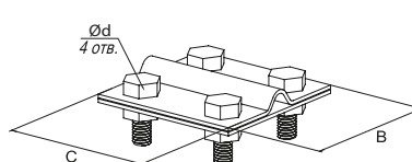
Зажим (полоса-прут)
