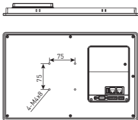
Рис. 4b – Размеры под крепление VESA для RSC-15E
