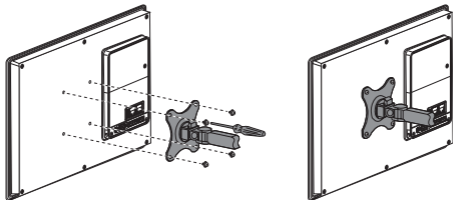
Рис. 6 - крепление с помощью кронштейна
