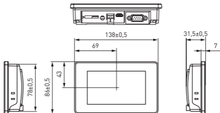
Рис. 1 – Габаритные размеры RSC-4
