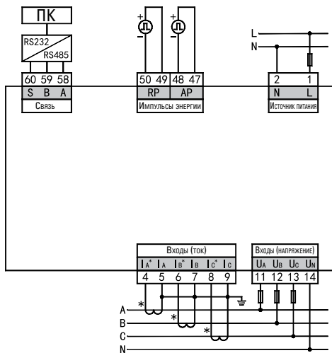
Рис. 4 Расположение клемм
