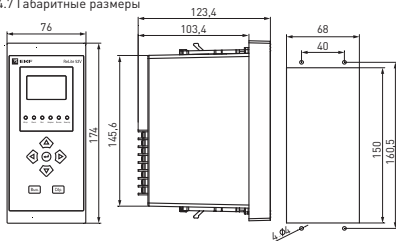
Рис. 3 – Габаритные размеры устройства ReLite 52 в вертикальном исполнении
