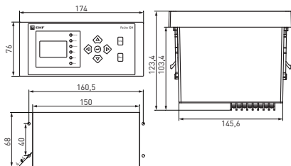
Рис. 4 – Габаритные размеры устройства ReLite 52 в горизонтальном исполнении
