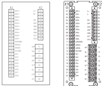
Рис. 2 – Расположение клемм
