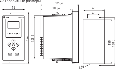
Рис. 3 – Габаритные размеры устройства ReLite 52 в вертикальном исполнении
