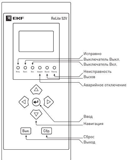
Рис. 1 – Лицевая панель ReLite 52
