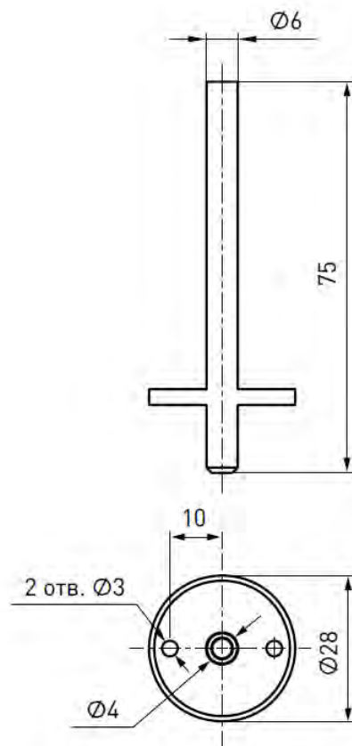
Штуцер
