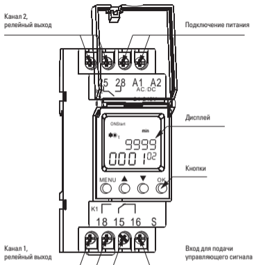
Рис.1 Таймер TM-24
