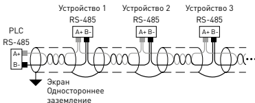
Рисунок 36 – Подключение интерфейса RS-485
