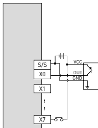
Входы: PNP-транзисторы
