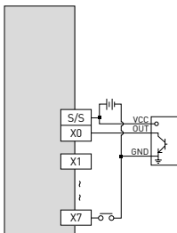
Входы: NPN-транзисторы
