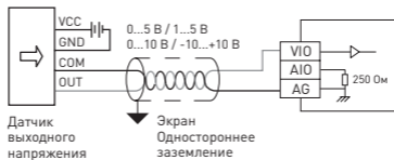
Рисунок 4 – Подключение аналоговых входов (входной сигнал – напряжение)
