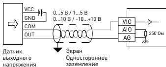
Рисунок 4 – Подключение аналоговых входов (входной сигнал – напряжение)
