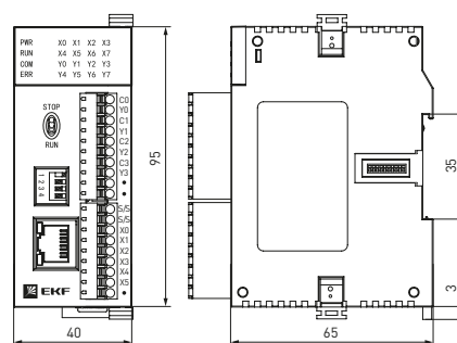
Контроллер PRO-Logic
