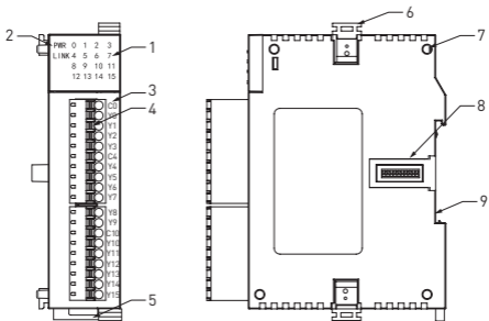
Рисунок 3 – Основные элементы модуля дискретного ввода/вывода
