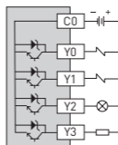
Выходы: NPN-транзисторы
