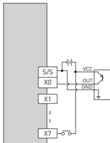
Входы: PNP-транзисторы
