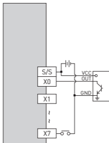
Входы: NPN-транзисторы
