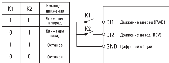
Рис. 6-6. Двухпроводной режим 1
