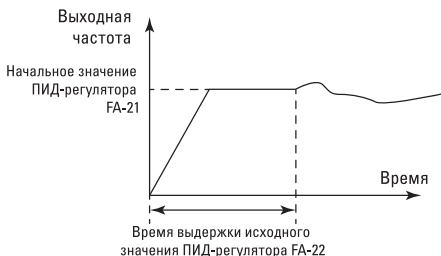
Рис. 6-28. Схема функции стартера ПИД-регулятора
