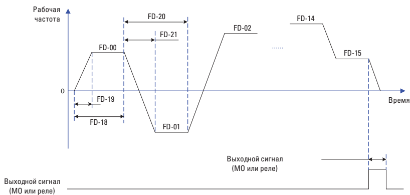
Схема работы простого ПЛК
