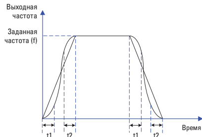
Картина А: схема S-кривой ускорения/торможения А
