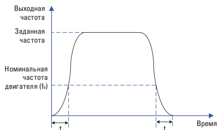
Картина В: схема S-кривой ускорения/торможения В
