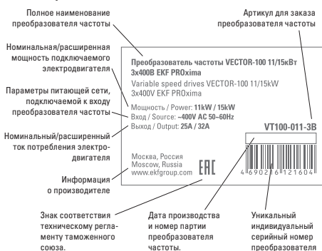
Рис. 2-2 Паспортная табличка.
