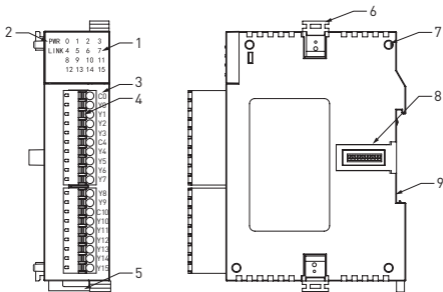
Рисунок 3 – Основные элементы модуля дискретного ввода/вывода
