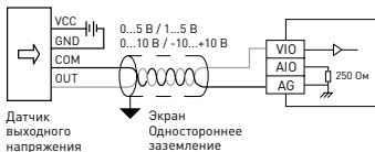
Рисунок 5 – Подключение аналоговых входов (входной сигнал – напряжение)
