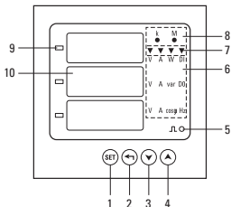
Рисунок 9 – Схема панели управления
