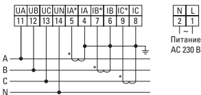
Рисунок 5 – Схема подключения прибора DMC
