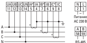
Рисунок 6 – Схема подключения прибора DMC-r
