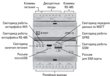
Рисунок 1. Внешний вид контроллера ePRO-6-4-230-W
