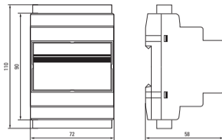
Рисунок 3 – Габаритные и установочные размеры
