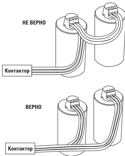
Рис. 3 – Параллельное подключение конденсаторов
