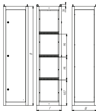
Рис.1 - Общий вид шкафов ВРУ-1 Unit S
