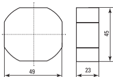
Рис. 4 Габаритные и установочные размеры
